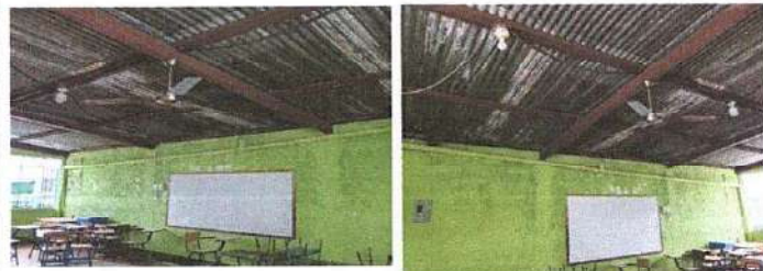
Foto 2: Sustitución de lámina, por lámina troquelada aluzinc calibre 26 y repacación de canal
