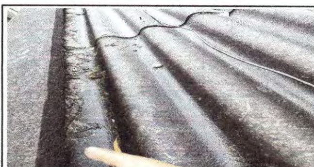
Foto 24: Filtración en laminas en las orillas de lado afuera, mantenimiento para lámina galvanizada para capotas.
