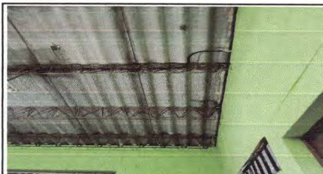
Foto 22: Baño de varones cambio de láminas quebradas
