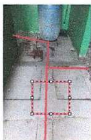
Foto 1: Piso de los Sanitarios lugar a nivelar y a colocar tubo que se conectará a drenaje acá se iniciará (baños de niñas)
