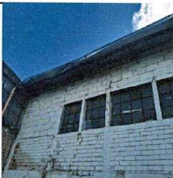
Foto 5: Desmontaje de canales del patio trasero e instalación de nuevos, con tres bajadas de agua para evitar la humedad.
