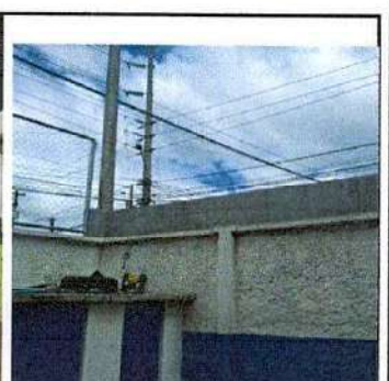
Foto 6: Repello y alisado en cocina, colocación de ventanas y balcones en cocina, ampliacion de muro perimetral.
