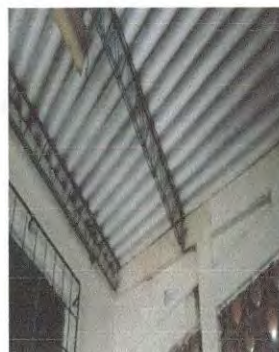
Foto 2: Cambio de lamina duralita por lamina alucink troquelada calibre 24 en 2 aulas, y pintar la estructura.
