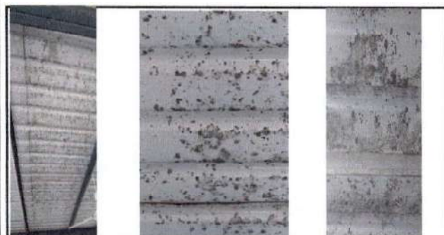
Foto 5: Sustitución de cubierta en modulo 1 de aulas
