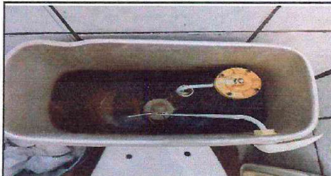
Foto 20: Sustitución de accesorios de inodoros (contra llave, tubo de abasto y tanque).
