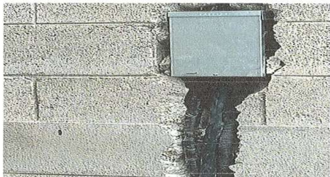
Foto25: INSTALACIÓN DE 3 TABLEROS ELÉCTRICOS CON SUS ACCESORIOS
