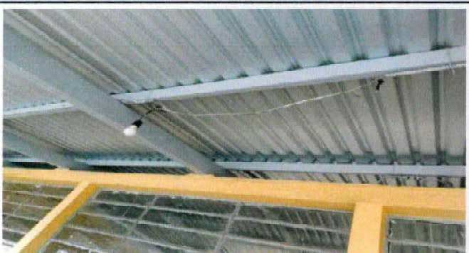
Foto 27: SUSTITUCIÓN DE CABLEADO ELECTRICO, INCLUYE DUCTO, CABLE ELÉCTRICO, CAJAS OCTAGONALES Y CAJAS RECTANGULARES, ABRAZADERA, TORNILLOS EN SALONES Y CORREDORES DE MÓDULO 2
