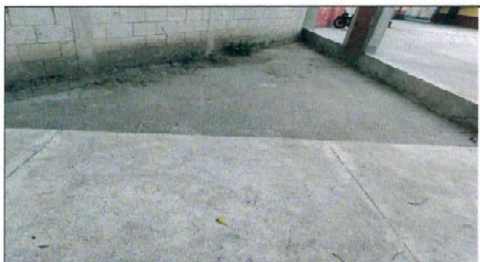
Foto 9: SUSTITUCIÓN Y FUNDICIÓN DE PISO DE CONCRETO CON 15 CMS DE ESPESOR INCLUYE ELECTROMALLA EN PATIO DELANTERO DE LA ESCUELA FRENTE A MÓDULO 1
