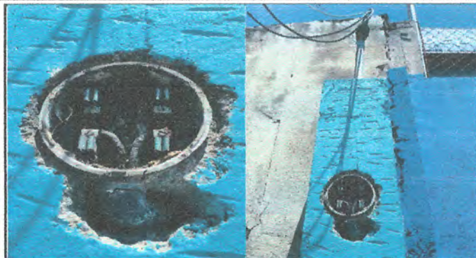
FOTO 1: Instalación de acometida, caja socket, tubo y mufa, demoler y fundir
