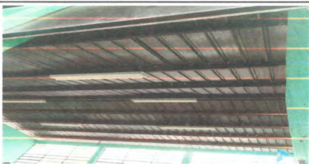
Foto 11: se tiene previsto cambio de lámina por lámina troquelada de aluzinc calibre 26 y mantenimiento de estructura de techo en aula de segundo primaria
