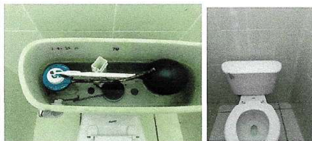
Foto 6: Se realizara el cambio de 8 kit de accesorios para tanques, en los sanitarios, sustitucion de mangueras, bridas y elementos de fijacion.
