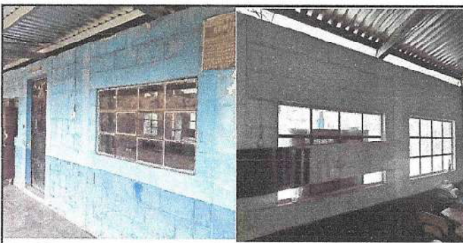
Foto 5: VENTANAS. Sustitución de ventanas de metal por ventanas de pvc blanco de 80mm y vidrio claro de 6mm con medidas de 1.66 mt de largo por 0.85mt de alto.
