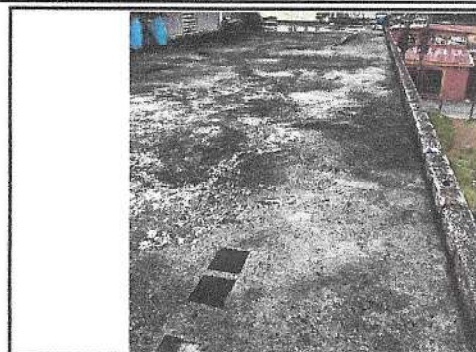
Foto 2: Deterioro de mezcón existente por los años de construcción y por lo tanto hay filtración de humedad en algunas partes de la losa.
