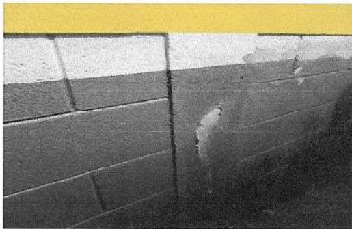
Foto 3: Colocación de azulejo por humedad.
