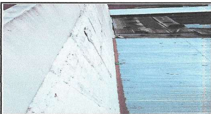
Foto 4: Limpieza, repello en muro y aplicación de impermeabilizante de pared externa de escuela de 15.40 de largo x 5 de alto
