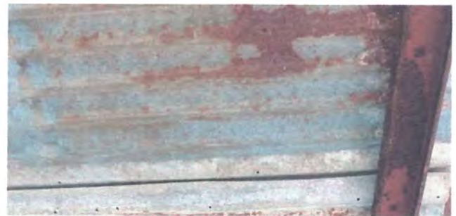
Foto 6: ESTRUCTURA DE TECHO- Bodega que se utilizará como salón, posee escasa estructura y deteriorada.
