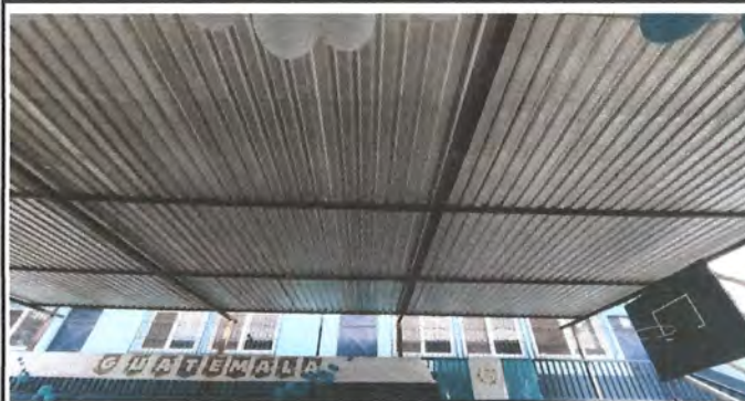
Foto 4: 1.1 Sustitucion de lamina, por lamina troquelada aluzinc calibre 26.
