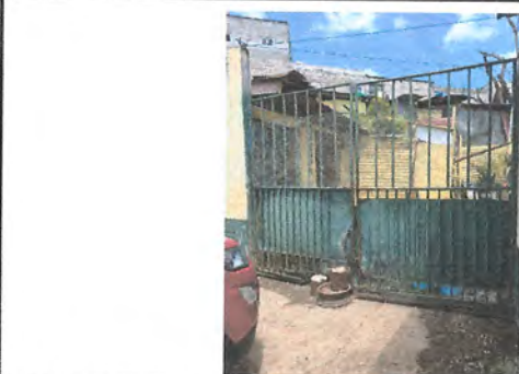
Foto 3: 12.1 REPARACION DE PORTON EN AREA DE GUARDIANA, INCLUYE SUSTITUIR TUBOS INFERIORES, INCORPORACION DE PASADOR, SUSTITUCION DE LAMINA Y PINTURA
