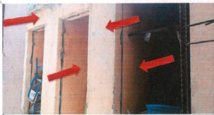
Foto 29: Instalación de azulejo similar a los existentes en el área de servicios sanitarios que se encuentran en la parte de atrás de una aula, el azulejo estará de piso a cielo, se incluye materiales y mano de obra.
