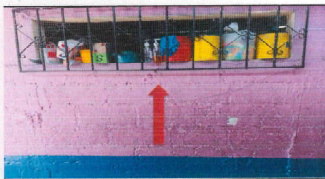
Foto 18: Romper pared para crear vano para ventanas de 03 aulas en un área de 1.50 de ancho x 1.00 de altura para dejar un dintel de 1.20 metros. Se resanará y tallará el área para dejar el vano listo para instalar ventana de PVC. Incluye materiales y mano de obra.
