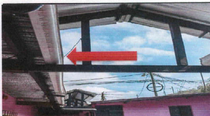
Foto 4: Desmontaje de lámina ondulada y canal de PVC blanco existente en el frente del área de aulas, incluye materiales y mano de obra
