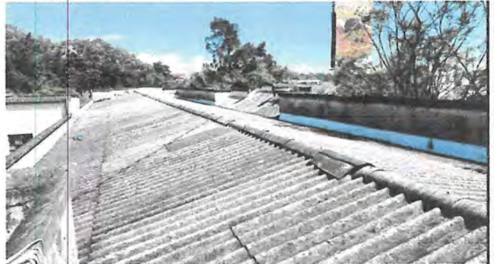
Foto 2: Sustitución de lamina duralita por lamina aluzinc calibre 26 en área frontal de segundo nivel de escuela de 315.95 mts cuadrados.
