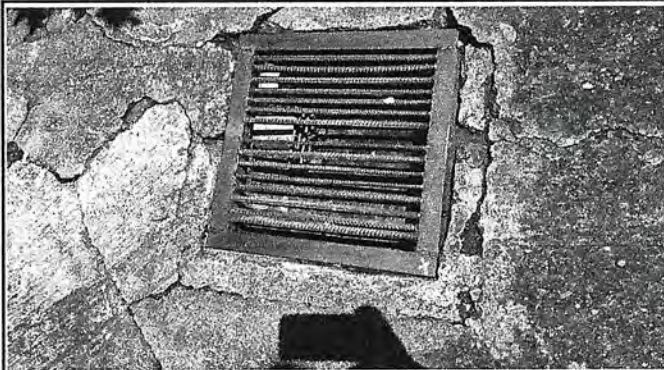
Foto 3: Sistema de drenaje con un deterioro significativo por la cantidad de agua pluvial.
