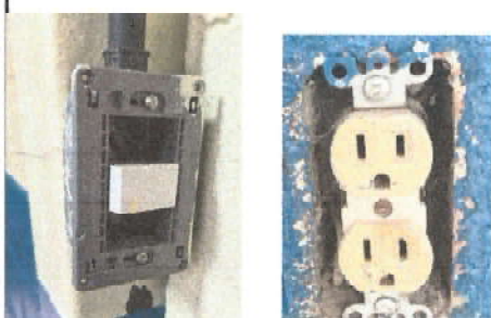
Foto 3: Instalacion de unidades de fuerza (tomacorrientes) incluye cable electrico en aulas de escuela.
