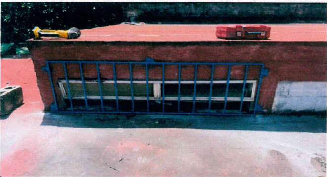
Foto 3: Sustitución de balcones de metal (en área de dirección de medidas de 1.90 mts por 0.55 mts de alto con hierro de 1/2 cuadrado)
