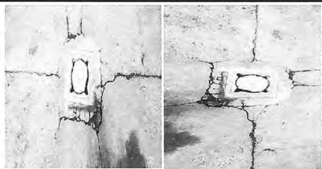
Foto7: sustitucion y modificacion de reposadera del patio en mal estado en el area de primaria.
