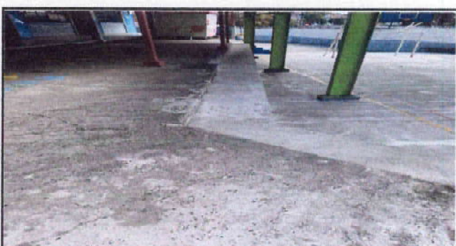
FABRICACIÓN DE BARANDA EN ORILLA DE CANCHA DEPORTIVA POR SEGURIDAD DE NIÑOS CON TUBO DE 1 1/2 CHAPA 18 Y TUBO DE 1 CHAPA 10 (CON SEPARACIÓN DE 10 CM)
