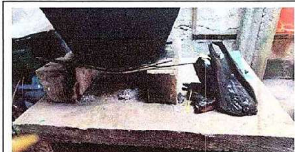
Foto 5: 20.2 Sustitución de estufa rural (completa) incluye chimenea y plancha de metal
