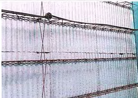
Foto 3: 2.3 Sustitución de estructura de soporte de metal, por metal.
