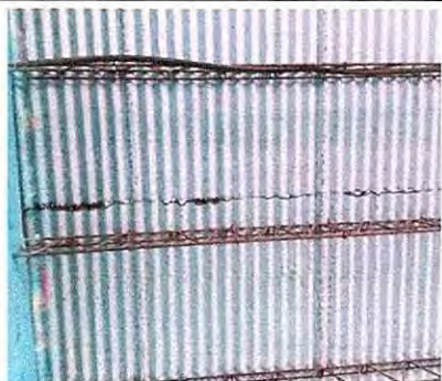
Foto1: 1.1. Sustitución de lámina por lámina troquelada aluzinc calibre 26
