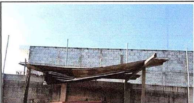
FOTO 3. ESTRUCTURA DE TECHO: 2.3 Sustitución de estructura de soporte madera, por metal
