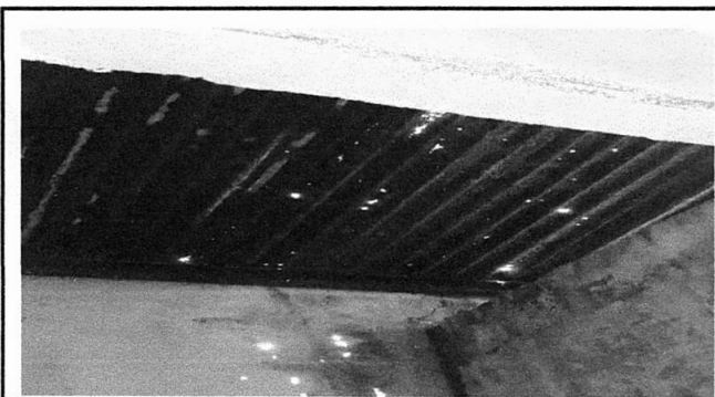
Foto 3: Sustrucción de lámina, por lámina troquelada aluzinc calibre 26. Módulo 5
