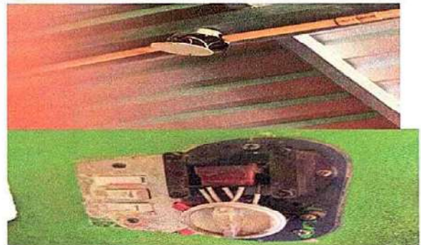
Foto 4: 19.11 Instalación de unidades luz (incluye interruptor, ducto y cable eléctrico)
