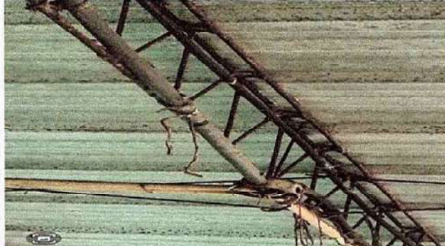
foto 4. 2 ESTRUCTURA DE TECHO. 2.1 Mantenimiento a estructura de soporte de metal.
