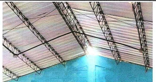
Foto 4: 1.2 Sustitución de capote existente dañado, por canal nuevo
