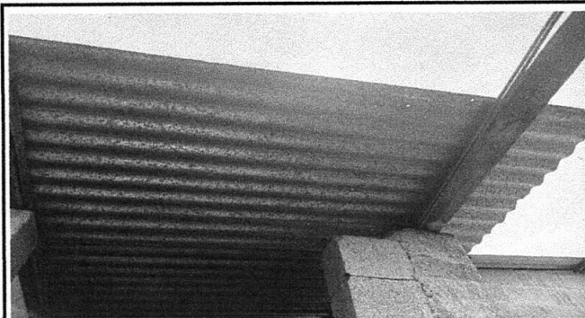
Foto1: 1.1 Sustitución de lámina, por lámina troquelada aluzinc calibre 26.
