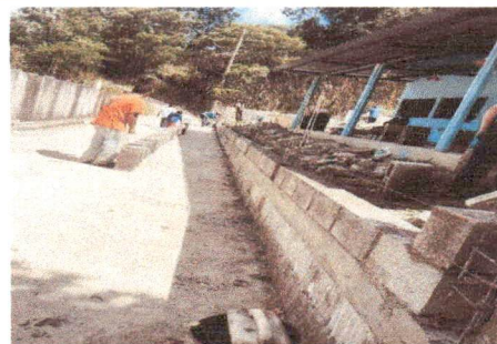
Foto 6: MUROS PERIMETRALES (REPARACIÓN DE MURO PERIMETRAL DE BLOCK CON TUBO H.C. Y MALLA GALVANIZADA Y SOLERAS INTERMEDIAS)
