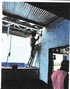
Foto1: Instalando lamina troquelada aluzinc calibre 26, mantenimiento de estructura de soporte de metal
