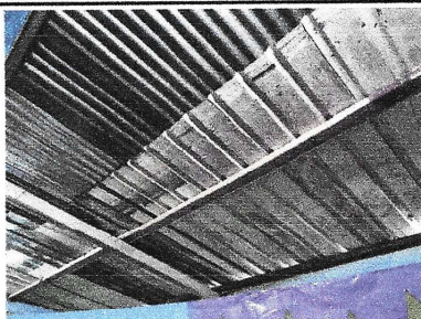
Foto 1: Sustrucción de lámina por lámina troquelada aluzinc calibre 26. Mantenimiento de estructura de soporte de metal.
