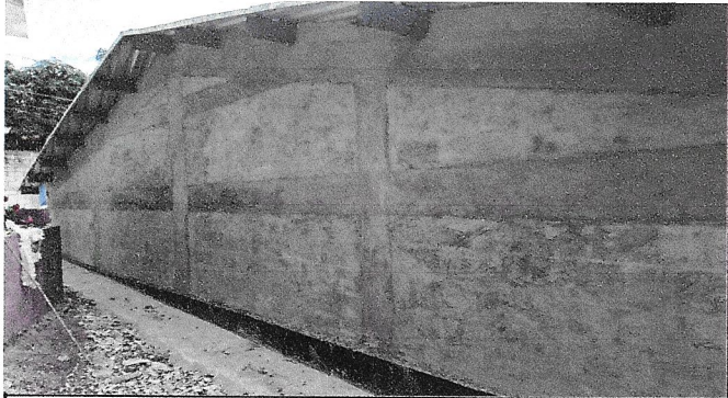
Foto1: Impermeabilización de muro colindante con el cementerio y drenaje francés para evitar la filtración del agua para los salones de clase.
