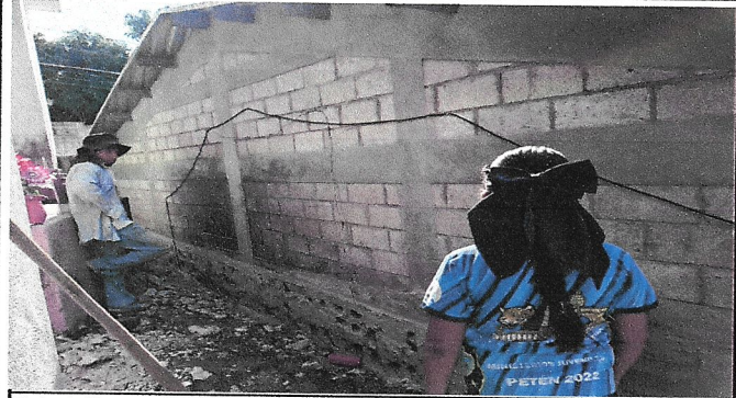
Foto 1: Excavación manual para impermeabilización e instalación de drenaje francés
