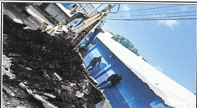
Foto 2: Excavación para impermeabilización de muro colindante con calle.
