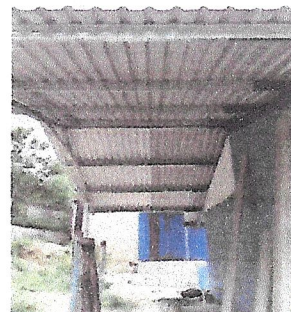
Foto 4: SUSTITUCION DE ESTRUCTURA DE MADERA POR ESTRUCTURA DE METAL
