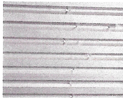
Foto 2: SUSTITUCIÓN DE LAMINA EN MAL ESTADO CALIBRE 26 POR LAMINA DE ALUCIN CALIBRE 24.
