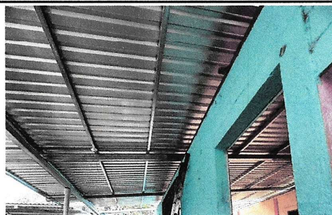
Foto 2: Sustitución de lámina, por lámina troquelada de aluzinc calibre 26
