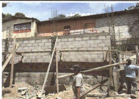
Foto 5: Reparación de muro perimetral
