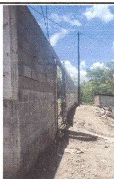
Foto 3: Continuación de losa de patio, instalación de pila prefabricada de dos lavaderos.
