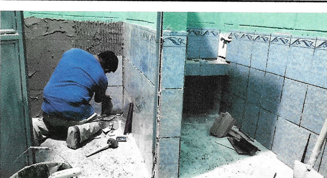
Foto 6: Reparación de Sanitarios
