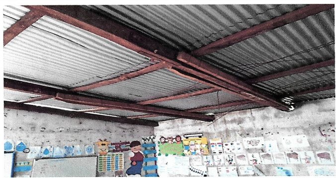
Foto 5: Sustitución de estructura de madera por estructura de metal.
