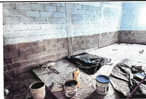
Imagen 4. instalación de piso de granito
