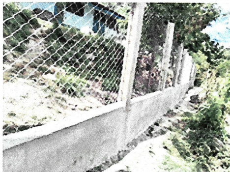
Foto 6: SEGUIMIENTO DE MURO EXISTENTE
