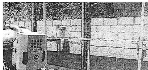
REPARACIÓN DE MURO PERIMETRAL, NO.1
