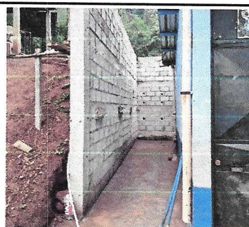
Foto 4: se muestra el muro desde un plano más cercano para apreciar con más precisión los detalles del muro de contención.
