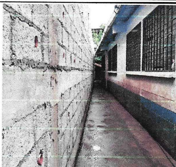
Foto 1: El muro ya se encuentra terminado, esta fotografía muestra la parte posterior de las aulas que se encontraban en riesgo
